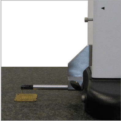
手表机芯高度测量
