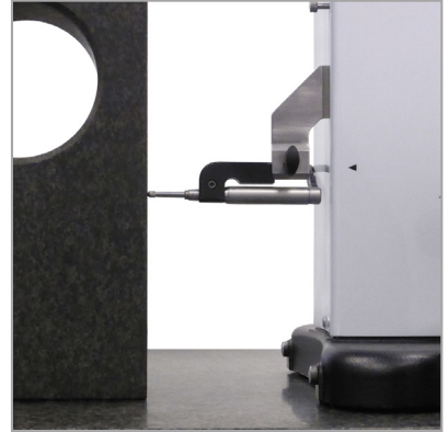
电子测头，测量垂直度
